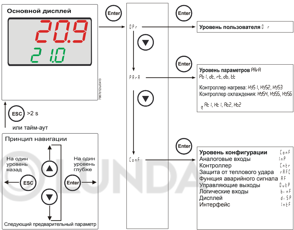
Иллюстрация 27: Конфигурация
