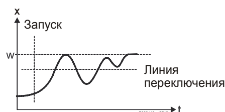
Иллюстрация 31: Значительная разница между фактическим значением и уставкой
