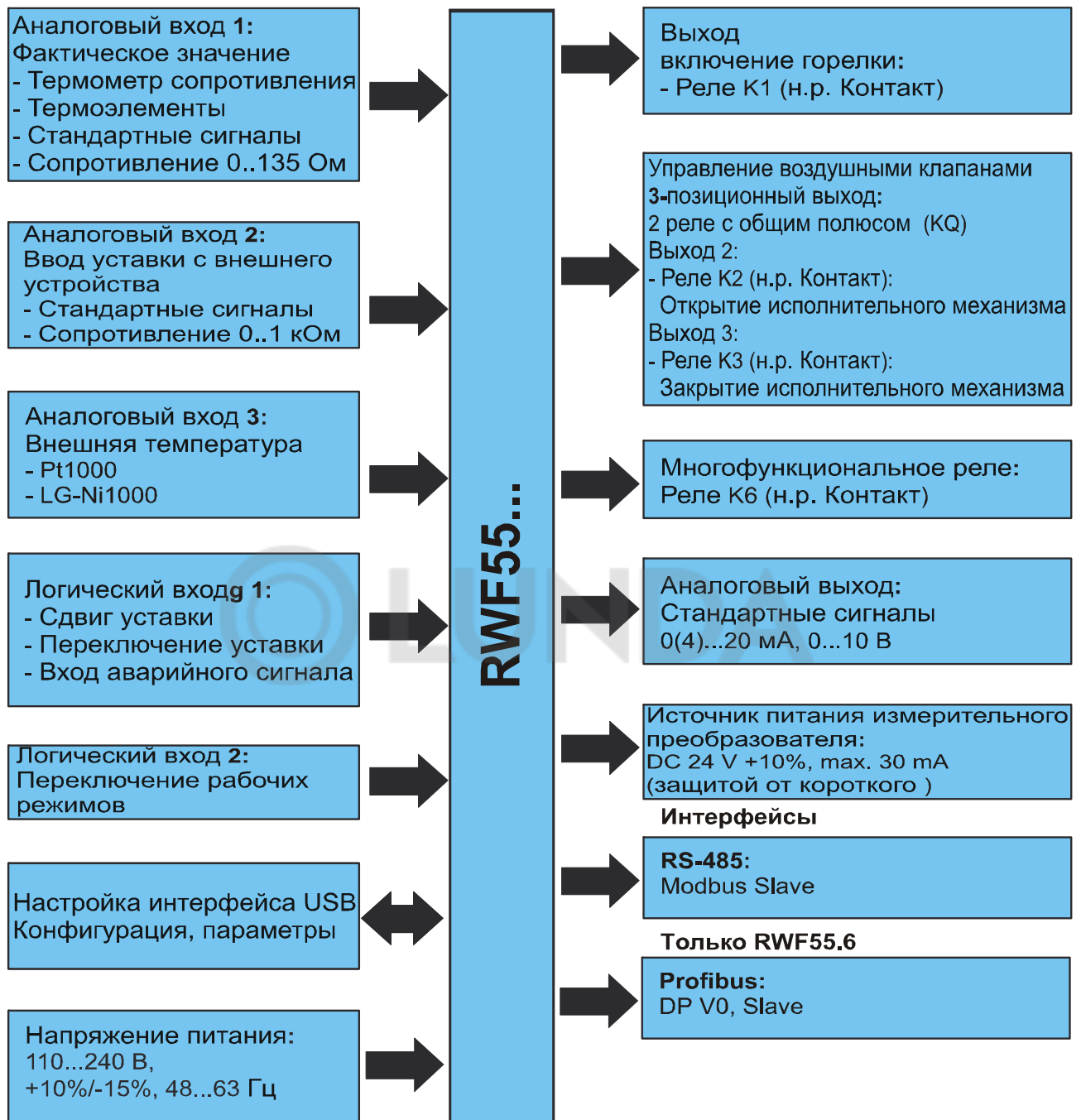
Иллюстрация 1: Блок-схема
