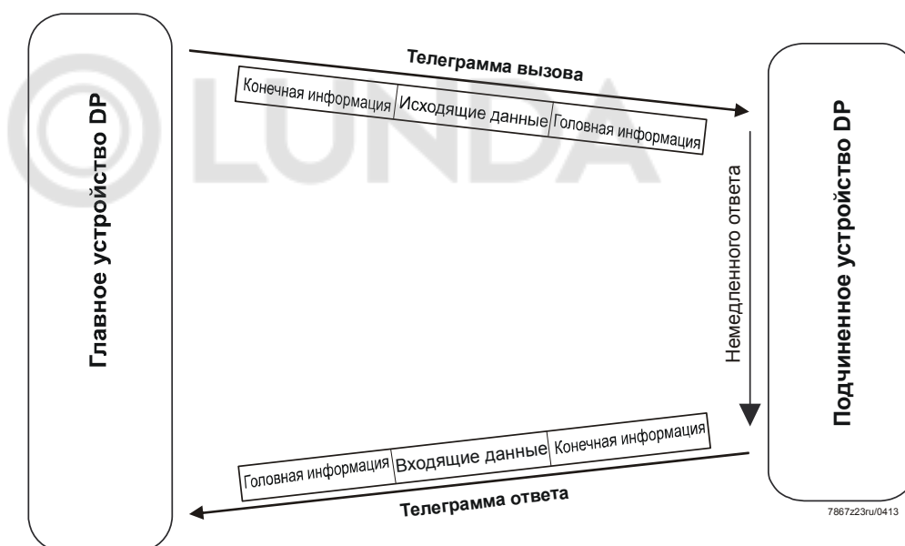
Иллюстрация 40: Передача полезных данных по шине Profibus-DP
