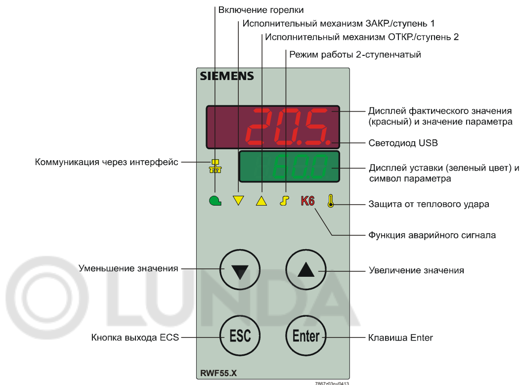
Иллюстрация 20: Пояснения к значению символов на дисплее и клавиш
