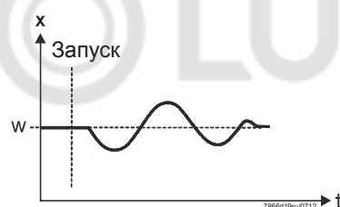
Иллюстрация 32: Малое отклонение регулируемой величины
