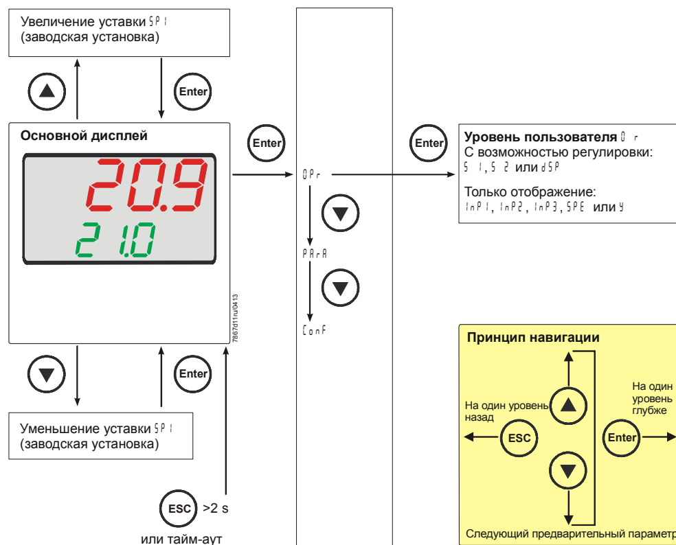
Иллюстрация 22: Основной дисплей
