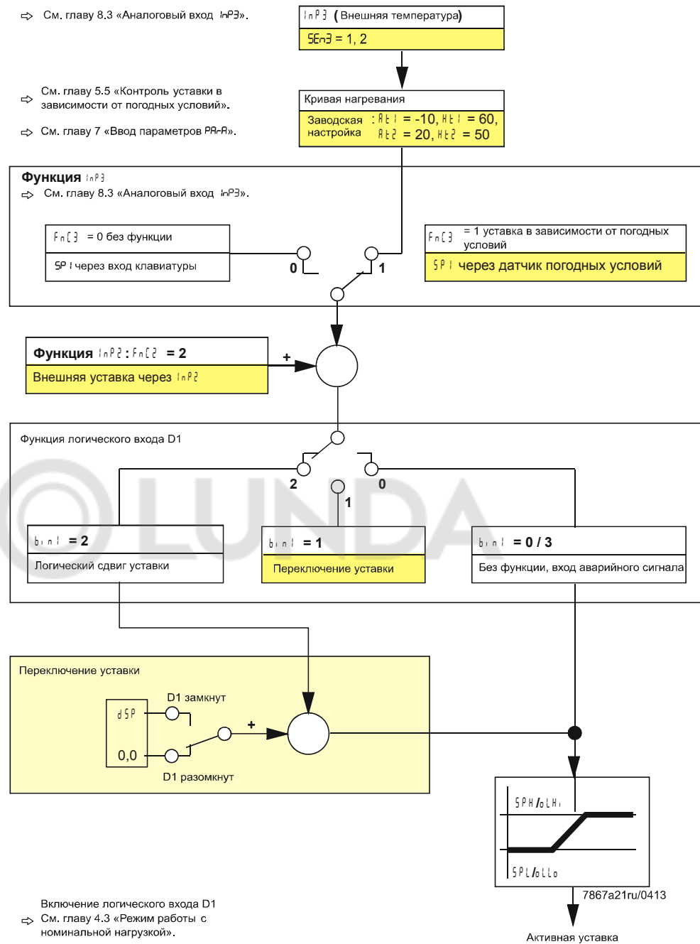
График 14: Сдвиг уставки аналоговый/логический
