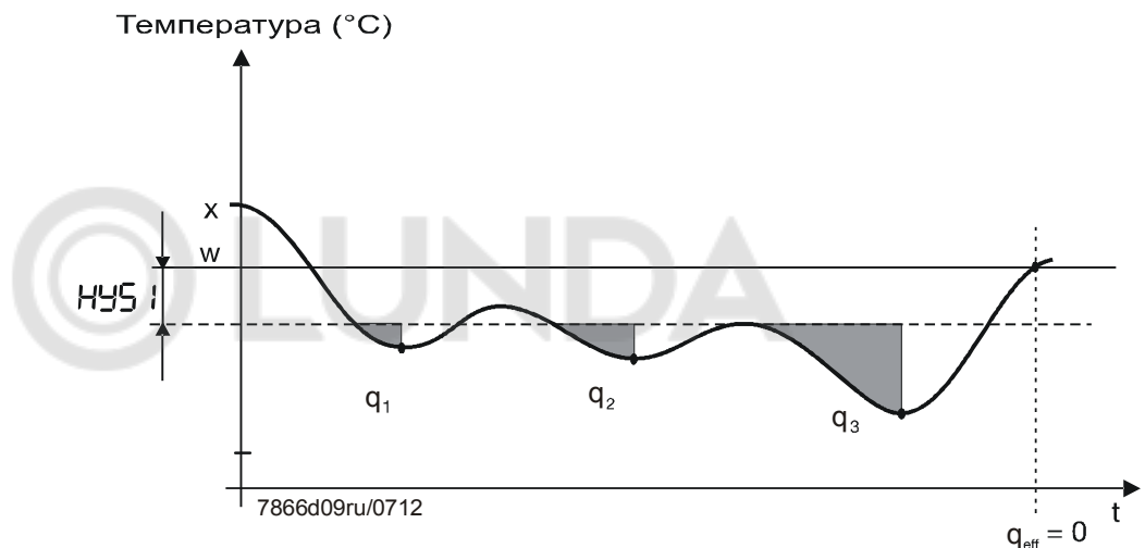
Иллюстрация 17: Программируемый цикл горелки, порог срабатывания (q)
