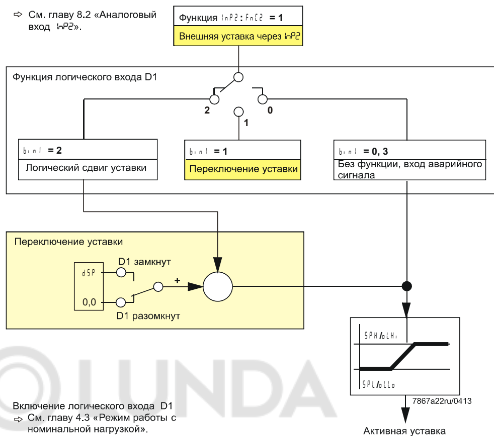
График 15: Внешняя уставка, логический сдвиг уставки через dSP
