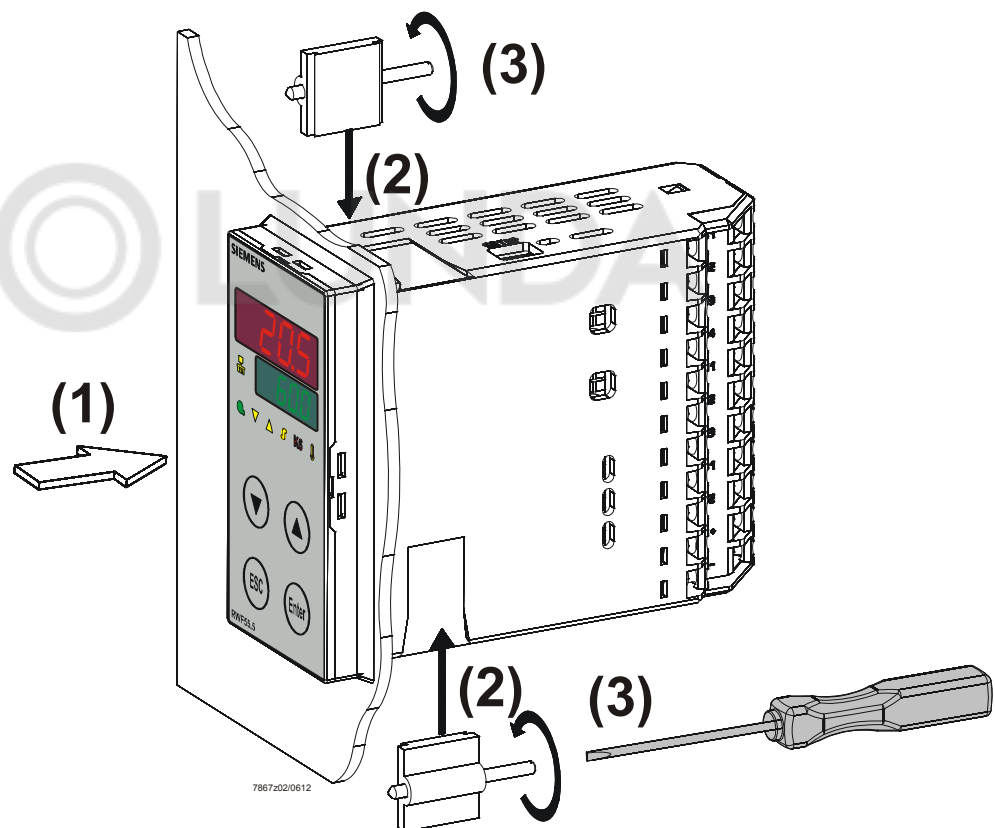
Иллюстрация 3: Установка в вырез панели управления
