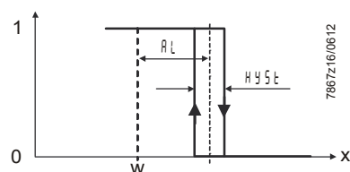
График 28: Функции аварийного сигнала Ik1 – Ik6
