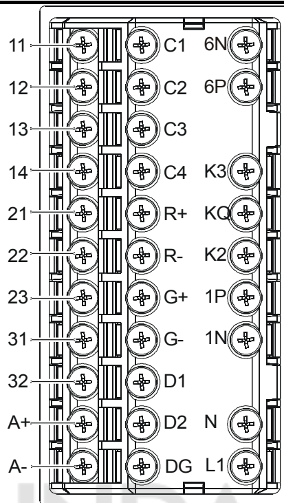
Иллюстрация 5: Назначение выводов
